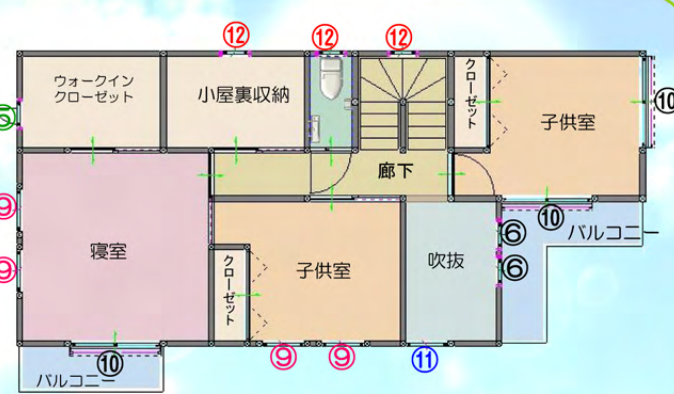
2階平面図
