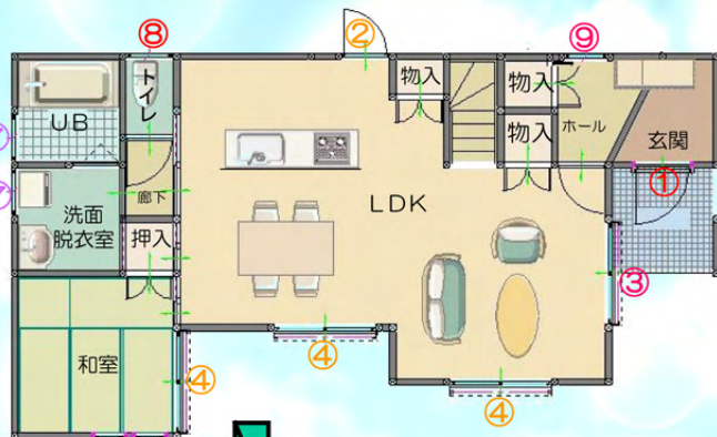
1階平面図
